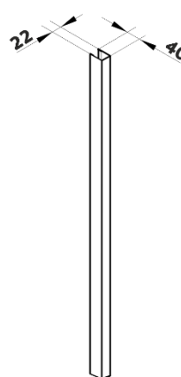
② Profil metallic de fixare pe stâlp U20
