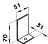
④ Colțar prindere beton
