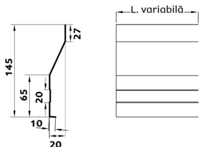
④ Colțar prindere beton
