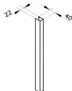
⑥ Capac închidere U20
