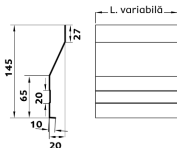
① Lamelă front 65
