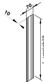
③ Capac riglă rigidizare
