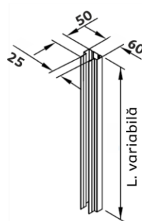
⑤ Profil metalic de fixare pe stâlp 25
