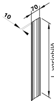
③ Capac riglă rigidizare
