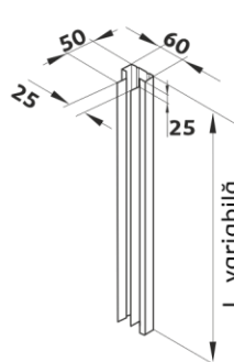
⑥ Capac închidere 25
