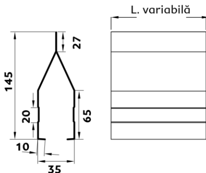
① Lamelă front 65
