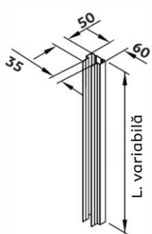
② Profil metallic de fixare pe stâlp 35
