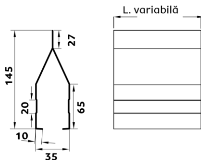
① Lamelă front 65
