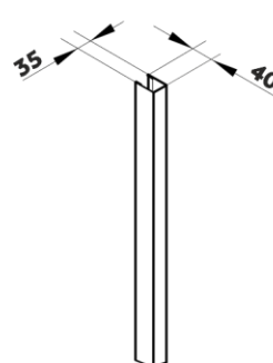
③ Capac închidere U35
